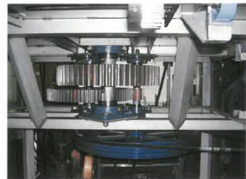
駆動部
