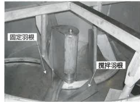
攪拌羽根
